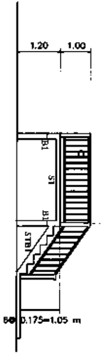
ราวบันได ไม้สูงราว 30x30 cm. (ดูแบบขยาย)
